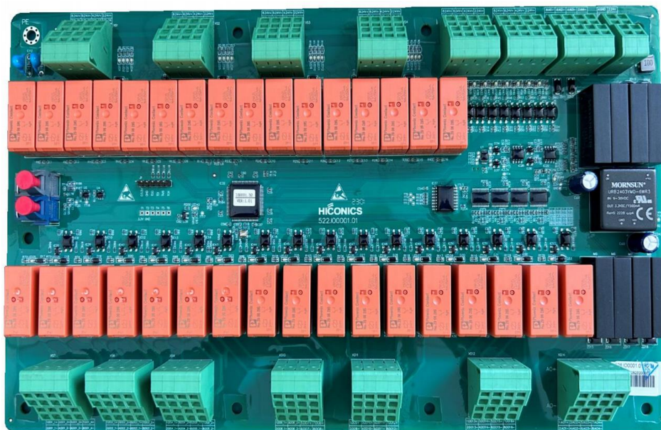
Рис. 1.13 – Плата вводов-выводов
