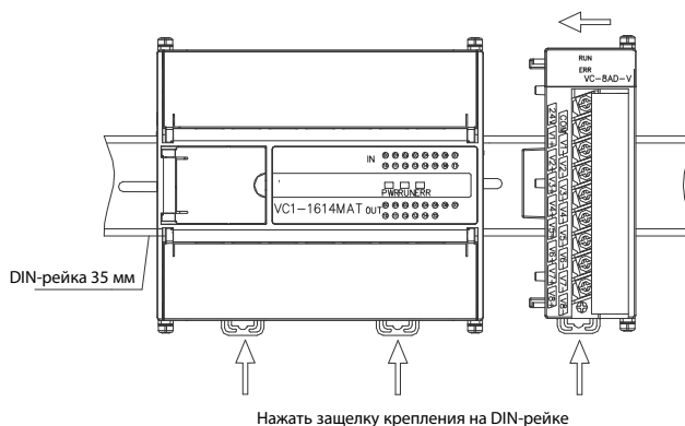
Рисунок 5-2 Установка модуля на DIN-рейку
