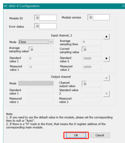
Рисунок 4-3 Пример стандартной настройки измерительного канала 3
