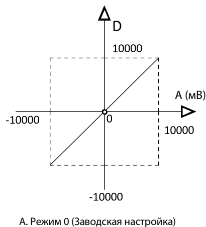
Рисунок 3-2. Изменение характеристики канала модуля VC-8AD-I
