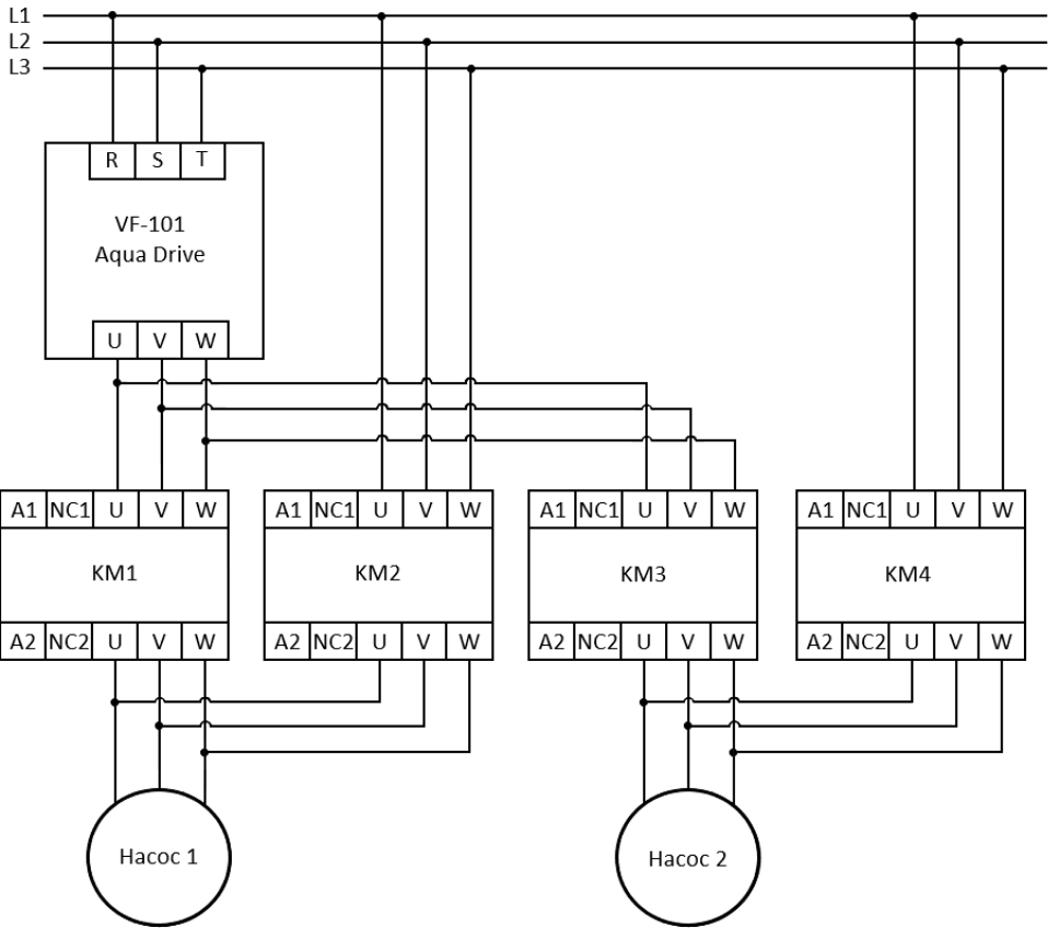
Рисунок 20 – Схема подключения силовой части каскадного регулирования (Одиночное управление)
