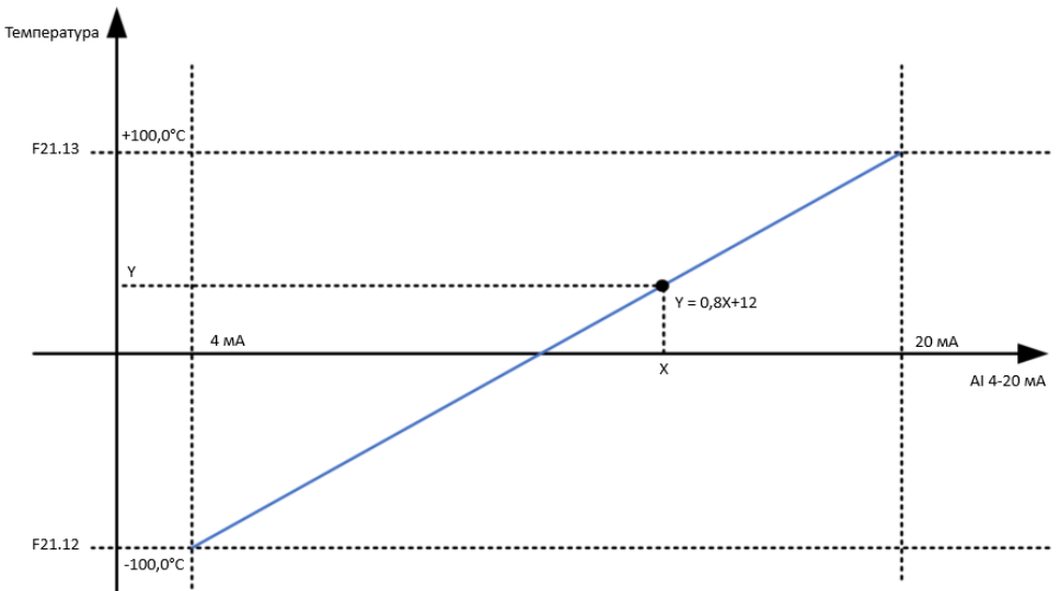
Рисунок 14 – Зависимость температуры и значения AI
