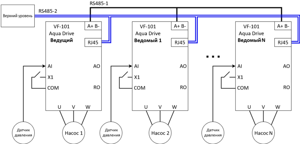
Рисунок 22 – Схема подключения для реализации каскадного регулирования (Групповое управление)
