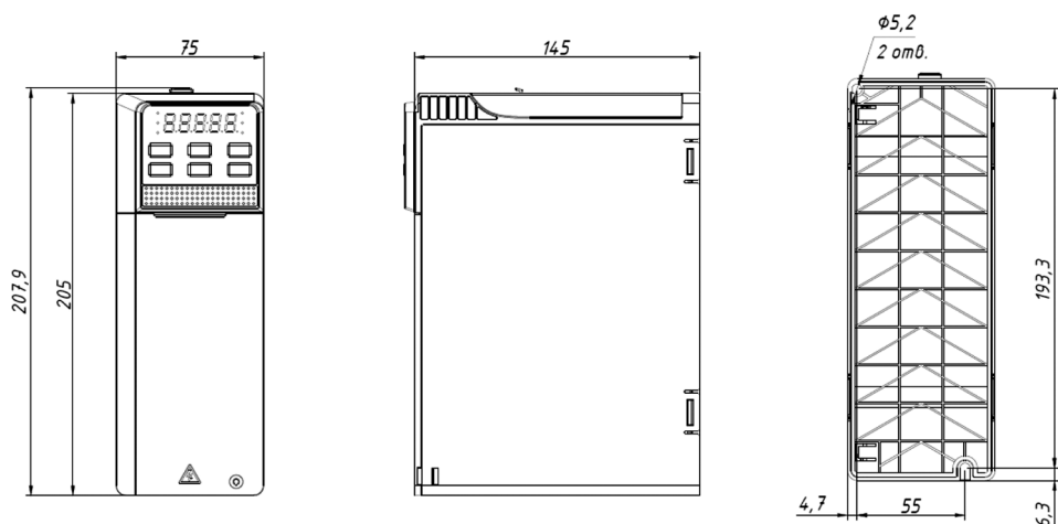
Рис. 3.6-2. Чертеж преобразователя частоты типоразмера C2
