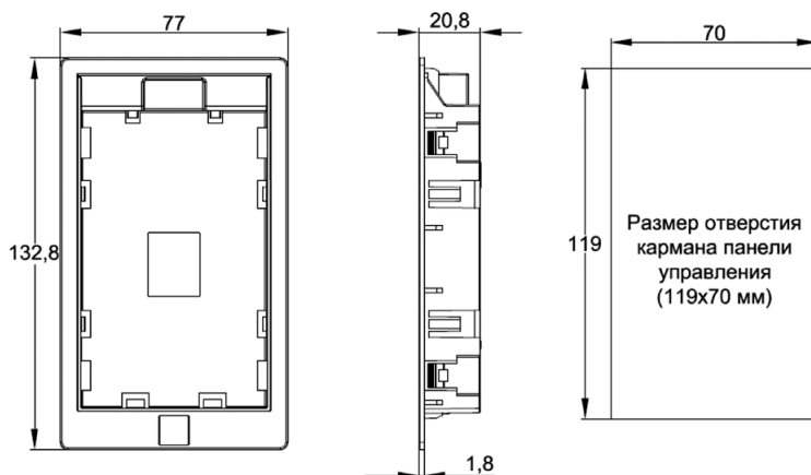
Рис. 3.7-2. Габаритные размеры держателя внешней цифровой двухстрочной панели управления (единица измерения – мм)
