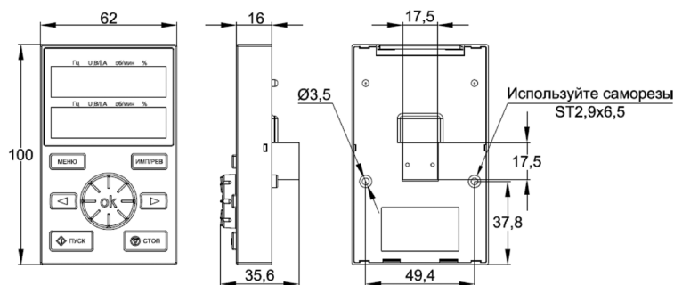
Рис. 3.7-1. Габаритные размеры и размеры отверстий внешней цифровой двухстрочной панели управления (единица измерения – мм)
