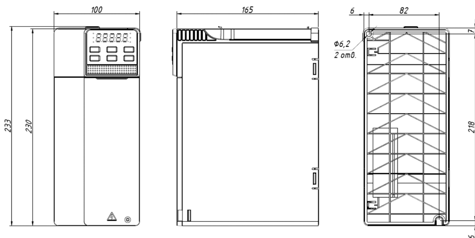
Рис. 3.6-3. Чертеж преобразователя частоты типоразмера C3
