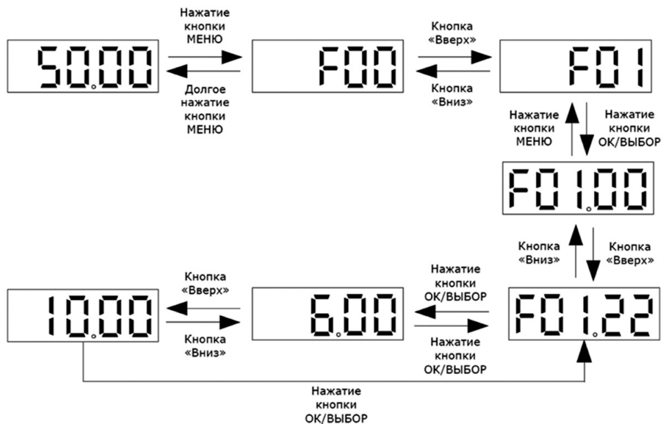
Рис. 7.1-2. Базовые операции с панелью управления
