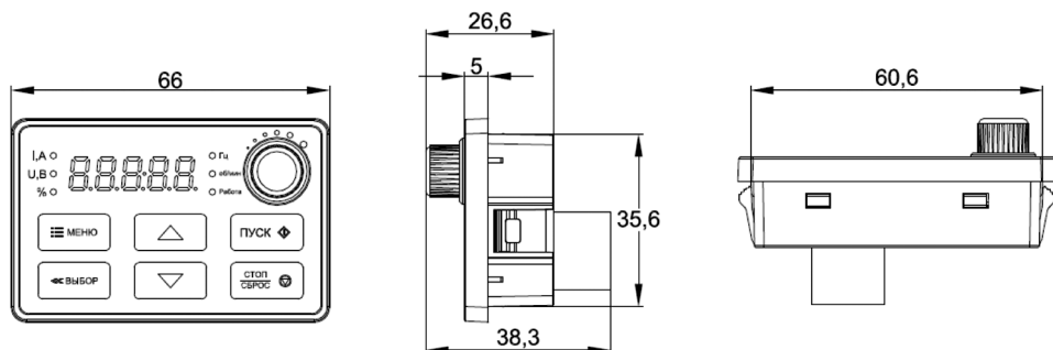
Рис. 3.7-3. Габаритные размеры и размеры отверстий внешней цифровой однострочной панели управления (единица измерения – мм)
