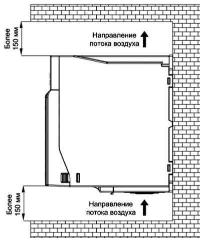
Рис. 3.5-1. Положение преобразователя частоты и требуемое пространство
