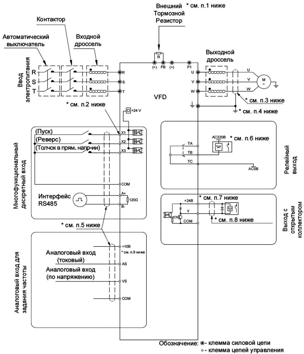
Рис. 4.2-1. Схема внешних подключений
