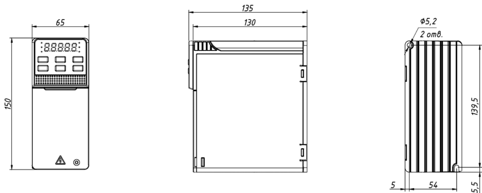
Рис. 3.6-1. Чертеж преобразователя частоты типоразмера C1
