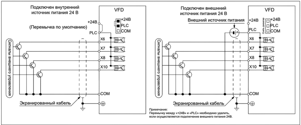
Рисунок 2.1-1. Подключение NPN
