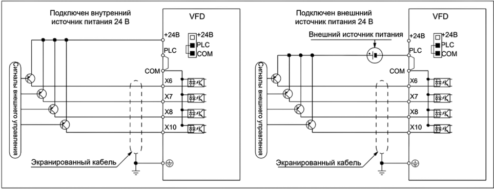
Рисунок 2.1-2. Подключение PNP
