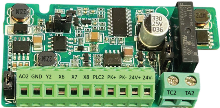
Рисунок 1-2. Внешний вид платы PBC00027
