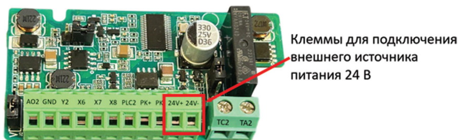
Рисунок 7-1. Подключение внешнего источника питания к PBC00027
