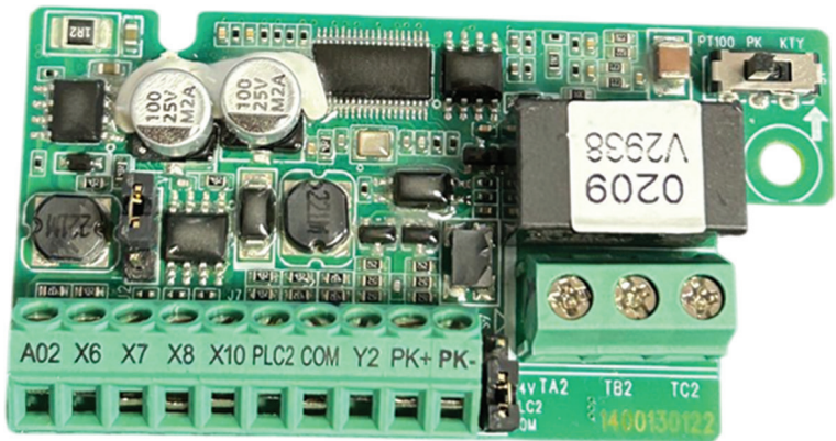
Рисунок 1-1. Внешний вид платы PBC00004
